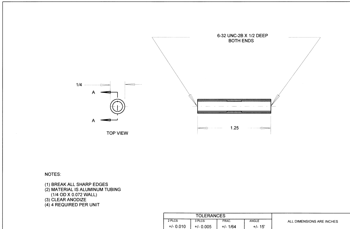
FIGURE L-9. 10-MICRON SPACER
